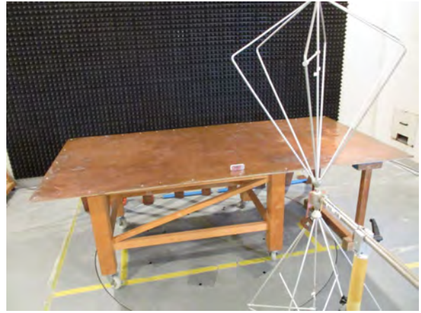
100 MHz-200 MHz (Vertical)
